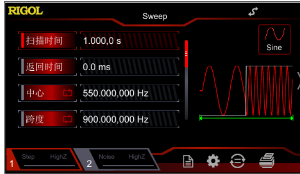
图 2-10 步进扫频
