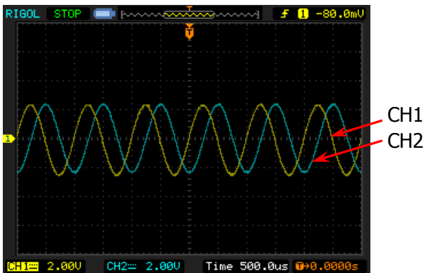
图 2-1 同相位前
