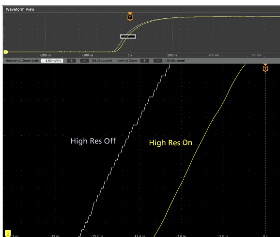
4 系列 MSO 的 12 位 ADC 及新型高分辨率模式实现了业界领先的垂直分辨率。
